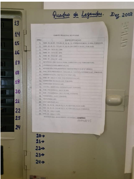
Foto 19 – Imagem do quadro de distribuição geral.
